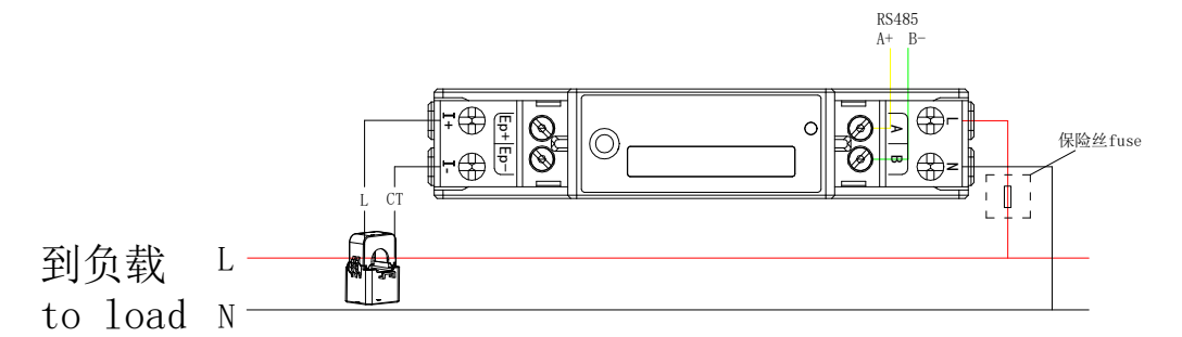
图 3 ADL200N-CT Figure 3 ADL200N-CT
