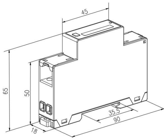
图 1 ADL200N-CT Figure 1 ADL200N-CT
